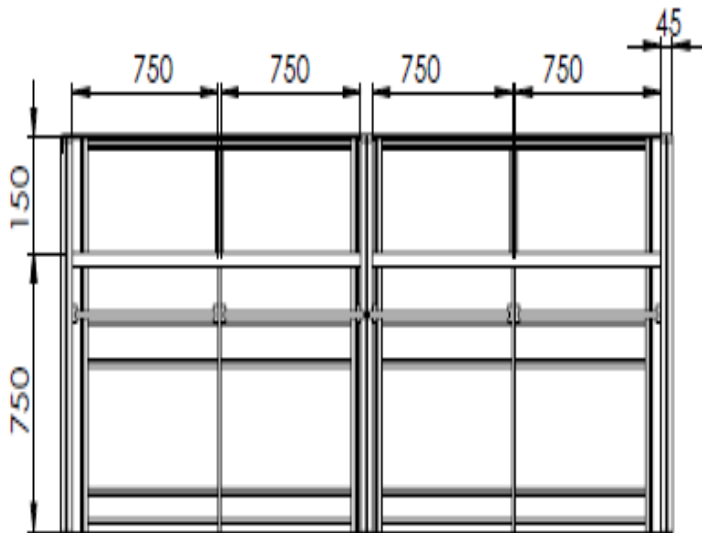
TOP ELEVATION
